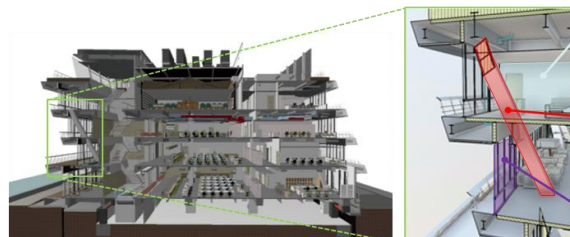
BIMモデル （建物全体）
