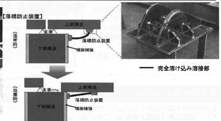
出典：落橋防止装置等の溶接不良に関する有識者委員会 中間報告書(H27.12.22) 34
